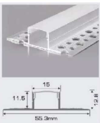
A15 - 2 D W55.3 x H12.8mm 156.000/m Nhôm định hình + Chụp nhựa PC
