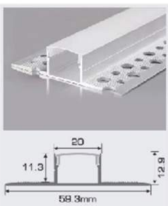
A20 - 2 D W58.3 x H12.9mm 176.000/m Nhôm định hình + Chụp nhựa PC
