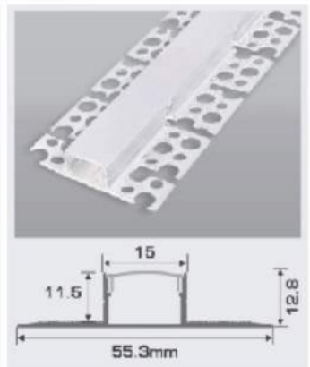
B15 - 2 D W55.3 x H12.8mm 236.000/m Nhôm định hình + Chụp nhựa Đẻo
