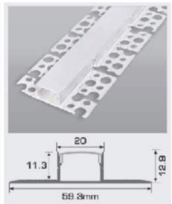
B20 - 2 D W59.3 x H12.9mm 256.000/m Nhôm định hình + Chụp nhựa Đẻo
