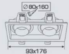
AFC 390/2 - MR16 (Không Bóng)
