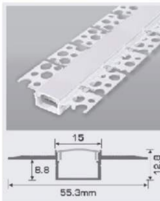
B15 - 2 T W55.3 x H12.8mm 236.000/m Nhôm định hình + Chụp nhựa Đẻo
