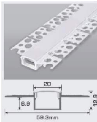
B20 - 2 T W59.3 x H12.9mm 256.000/m Nhôm định hình + Chụp nhựa Đẻo
