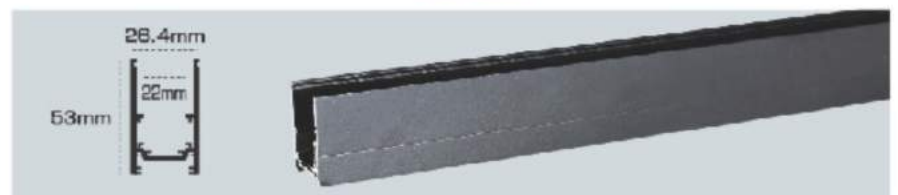
THANH RAY LẮP NỔI
