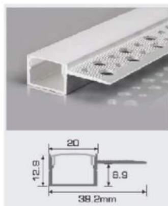
A20 - 1 T W38.2 x H12.9mm 156.000/m Nhôm định hình + Chụp nhựa PC
