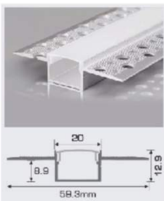
A20 - 2 T W58.3 x H12.9mm 176.000/m Nhôm định hình + Chụp nhựa PC
