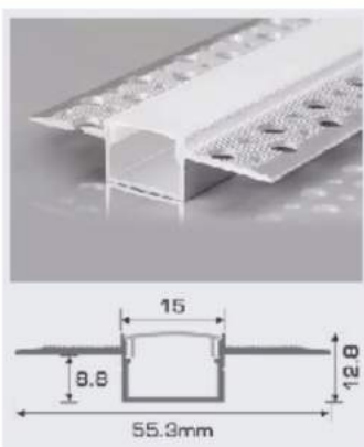
A15 - 2 T W55.3 x H12.8mm 156.000/m Nhôm định hình + Chụp nhựa PC
