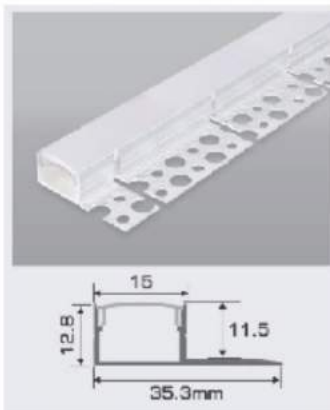
B15 - 1 D W35.3 x H12.8mm 216.000/m Nhôm định hình + Chụp nhựa Đẻo
