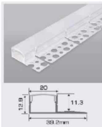
B20 - 1 D W39.2 x H12.9mm 236.000/m Nhôm định hình + Chụp nhựa Đẻo
