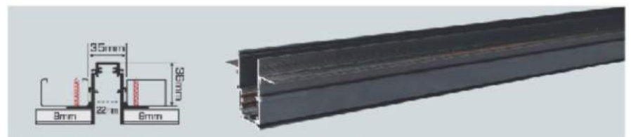
THANH RAY LẮP ẨM
