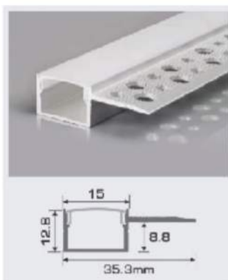
A15 - 1 T W35.3 x H12.8mm 136.000/m Nhôm định hình + Chụp nhựa PC
