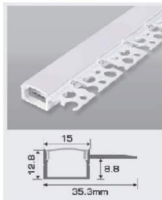
B15 - 1 T W35.3 x H12.8mm 216.000/m Nhôm định hình + Chụp nhựa Đẻo
