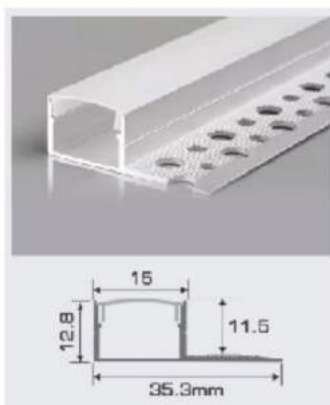
A15 - 1 D W35.3 x H12.8mm 136.000/m Nhôm định hình + Chụp nhựa PC
